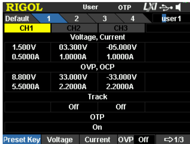
Рис. 0-21 Интерфейс пользовательских настроек
