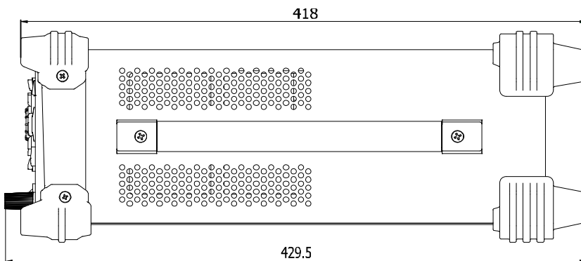
Рис. 0-2 Вид сбоку
