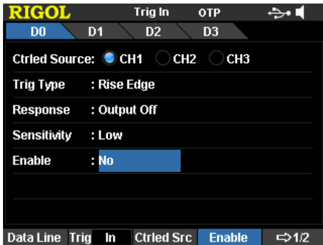
Рис. 0-9 Интерфейс настройки триггера
