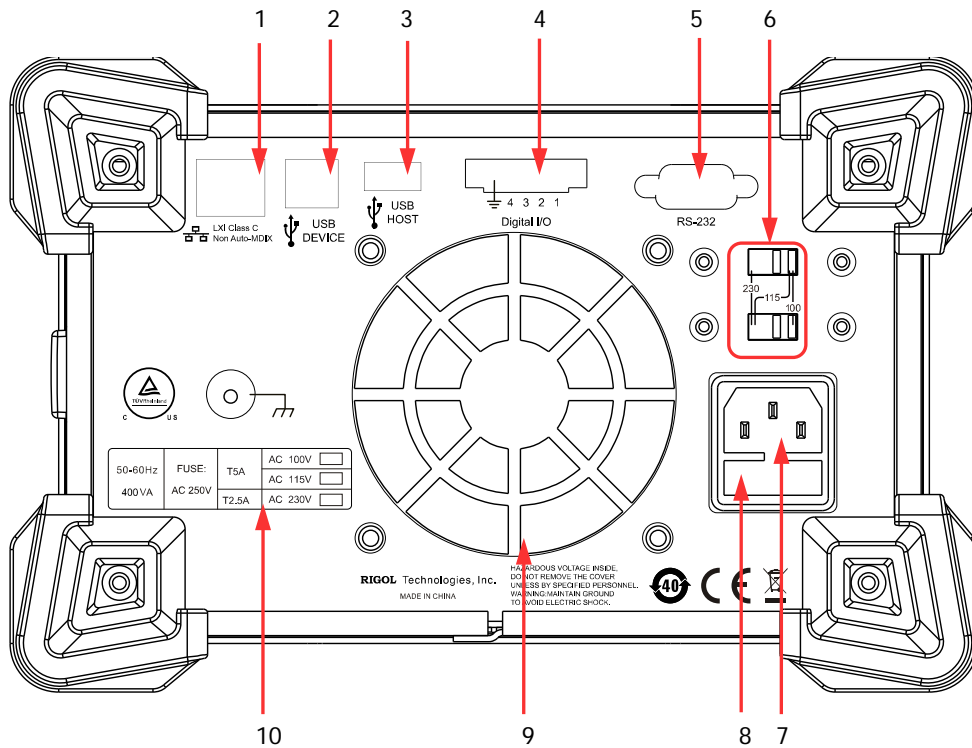
Рис. 0-4 Задняя панель DP831A
