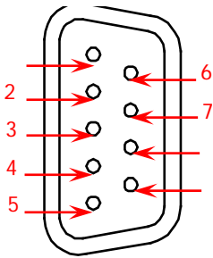
Разъем RS232
